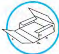
FEFCO_0401
